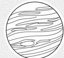
Neptune نبتون
