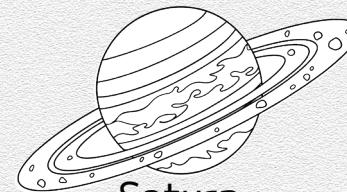
Saturn زحل
