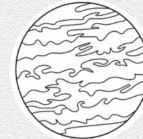
Venus الزهرة
