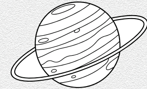
Uranus أورانوس
